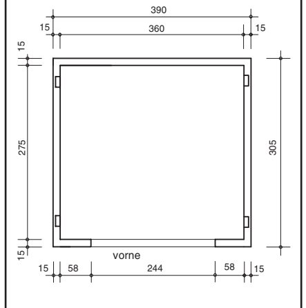
Grundriss Liftschacht
