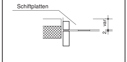
Detail Schiftplatten
