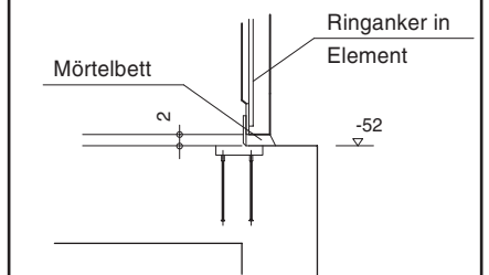
Detail Verankerung in Ortbeton X - X
